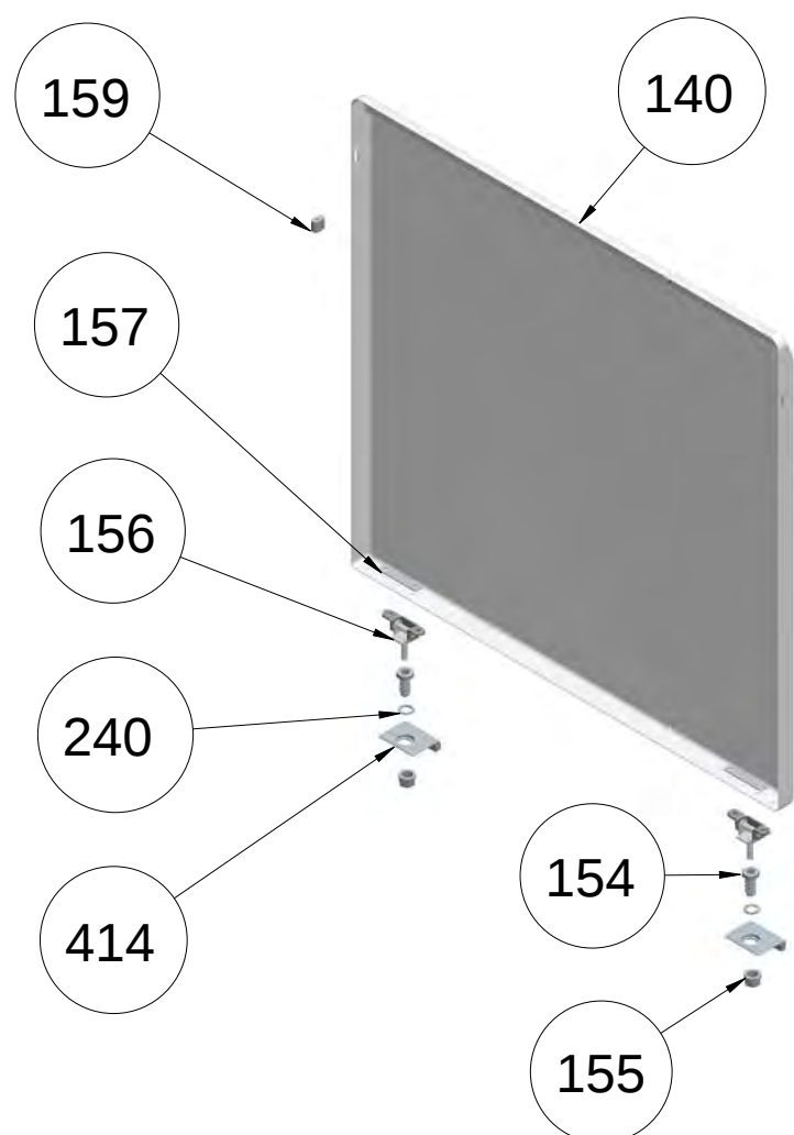
METAL LID OPTIONAL (POSITION NO 153)
